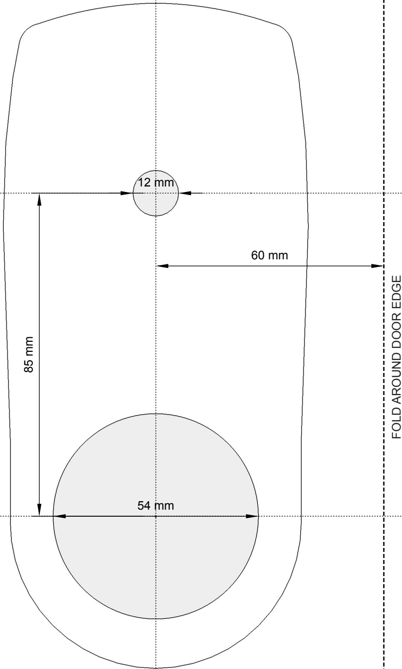
Remotelock 6i - 60mm backset template
