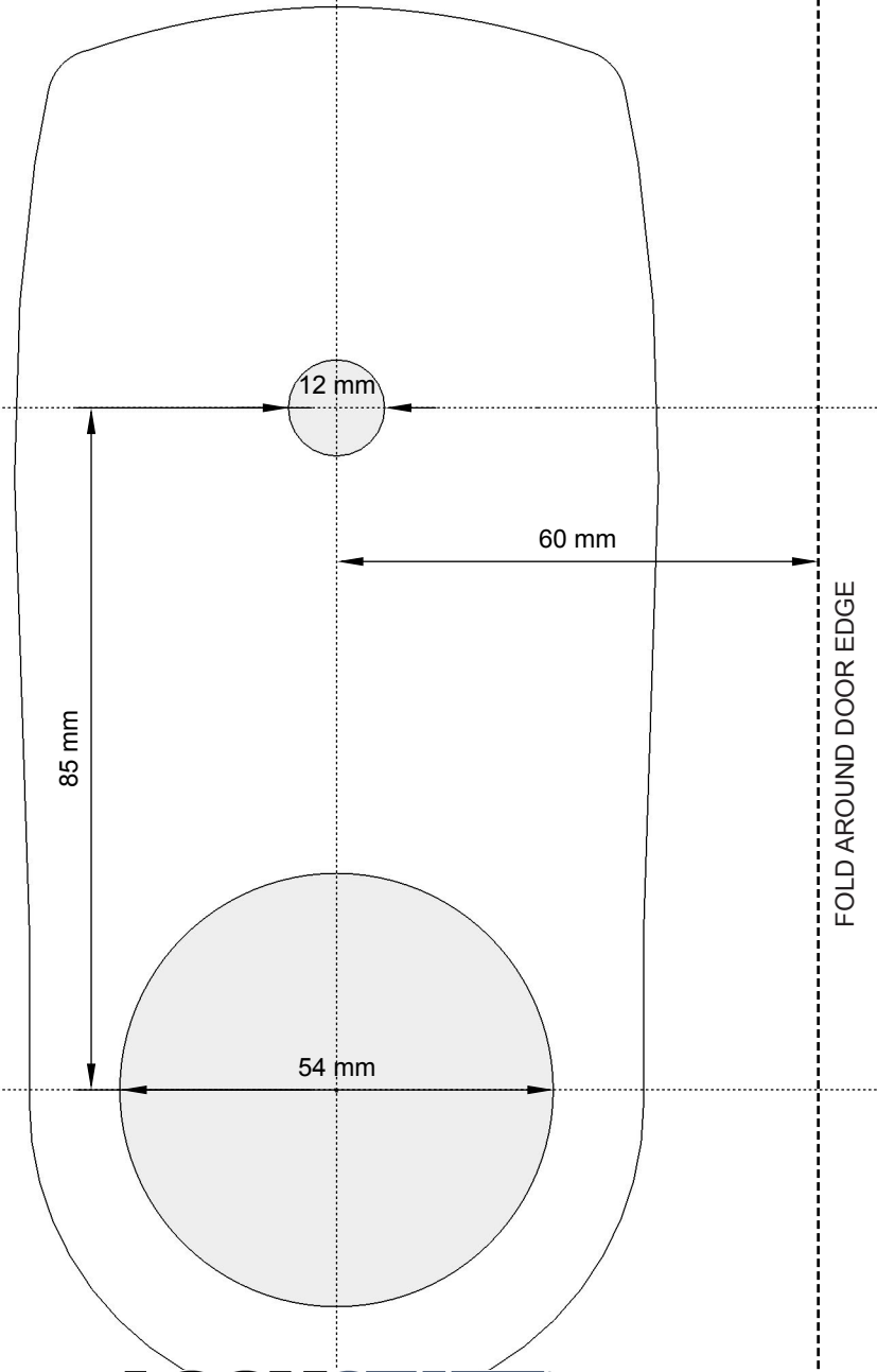
Remotelock 6i - 60mm backset template
