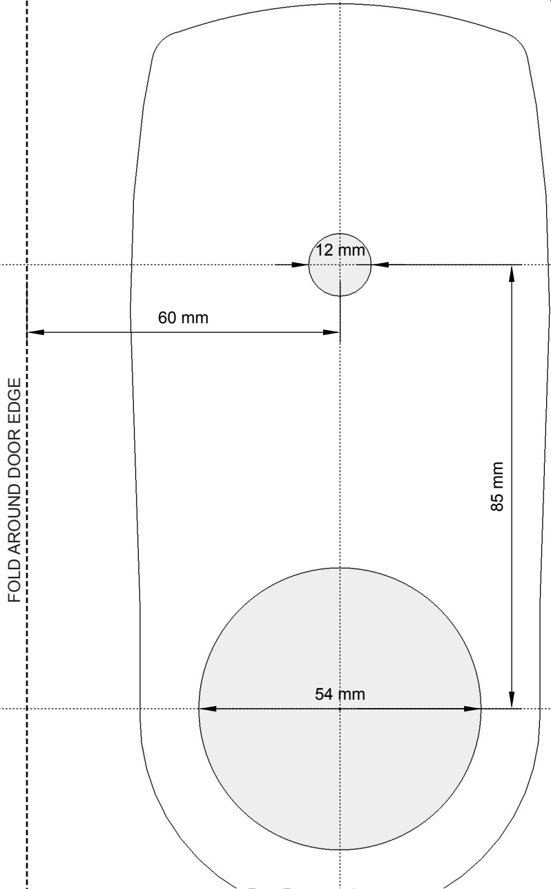
Remotelock 6i - 60mm backset template
